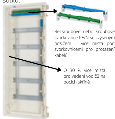
Obr. 1 Rozvodnice KLV v instalačním provedení
