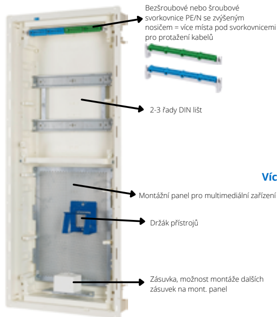
Obr. 3 Rozvodnice KLV v hybridním provedení
