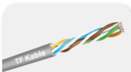
KABEL U/UTP-PVC-KAT5E 4×2×24AWG
