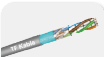
KABEL F/UTP-PVC-KAT5E 4×2×24AWG
