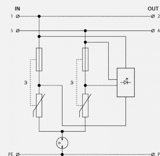
Schéma zapojení
