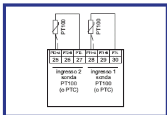
Schéma připojení tepelných snímačů typu PT100
