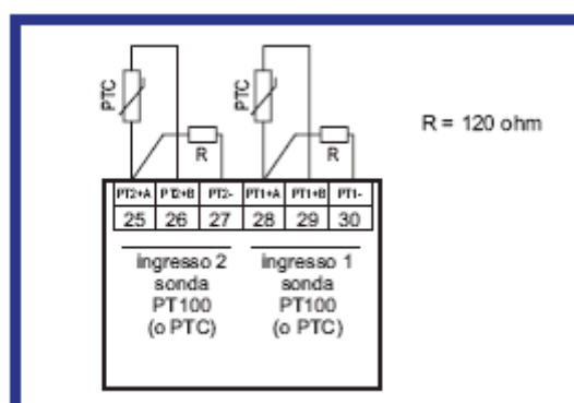
Schéma připojení tepelných snímačů typu PTC
