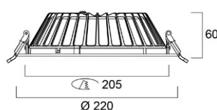
Insaver Slim 205
