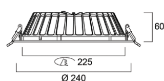
Insaver Slim 225
