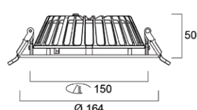
Insaver Slim 150
