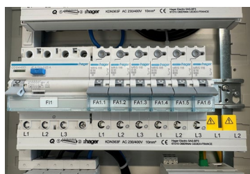
Jištění zásuvkových obvodů
