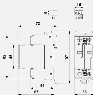
Rozměry
