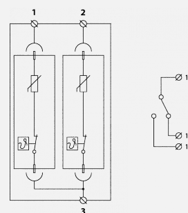
Schéma zapojení
