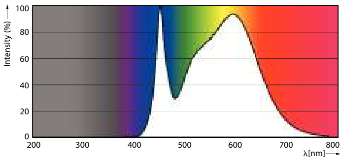
LEDlustre CorePro 7W P48 E27 840 FR-POC
