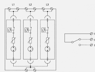
Schéma zapojení
