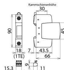
Rozměry DG S 48 FM
