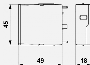
Rozměry
