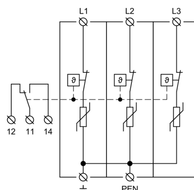
Vnitřní schéma zapojení
