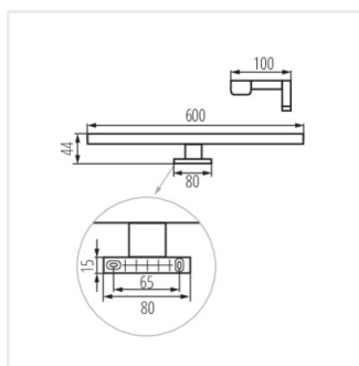
ASTIM IP44 12W-NW-C
