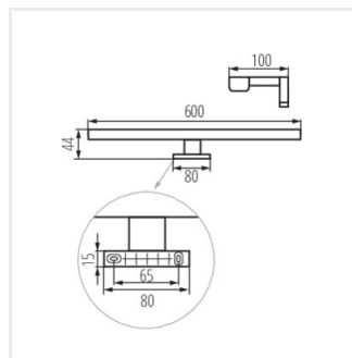
ASTIM IP44 12W
