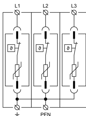
Vnitřní schéma zapojení
