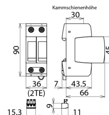
Rozměry DG M TT 2P 275 FM
