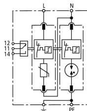
Schéma vnitřního zapojení DG M TT 2P 275 FM
