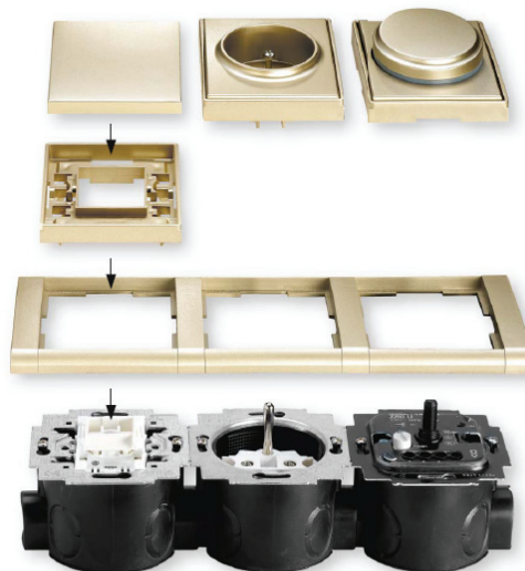
Obr. 3: Sestavování přístrojů s kryty a rámečky
