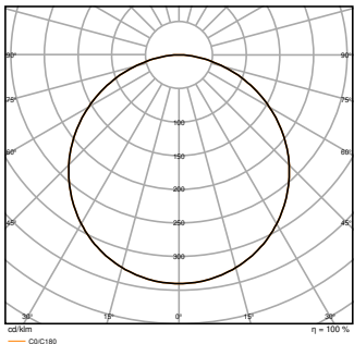
PL SF 1574 V 48W 940 U19 6240lm
