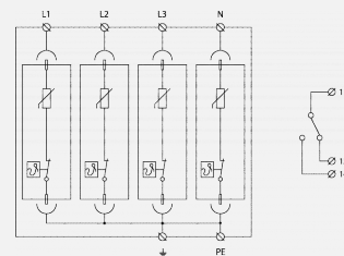
Schéma zapojení
