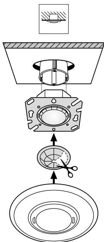
Zapuštěná montáž
