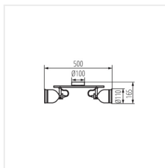
DERATO EL-2I
