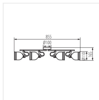
DERATO EL-4I
