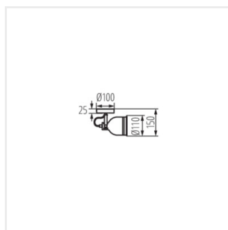
DERATO EL-10
