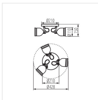
DERATO EL-3O
