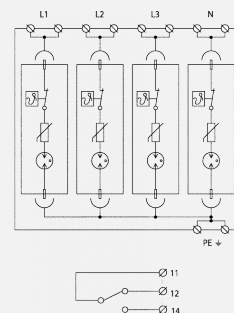
Schéma zapojení
