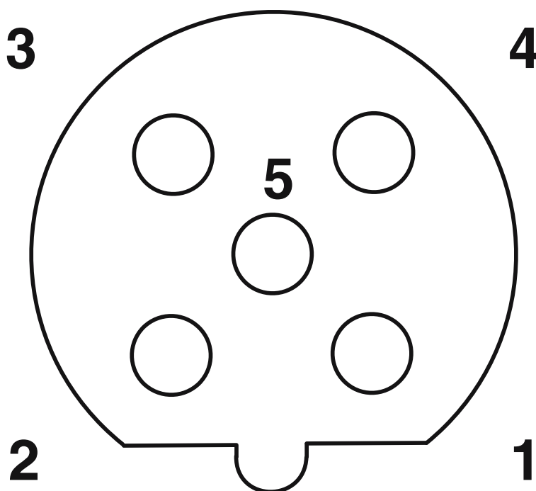
Schématický výkres
