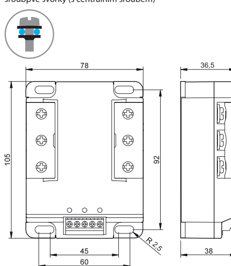
Typ 77.x3 šroubové svorky (s centrálním šroubem)
