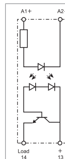
principiální schéma
