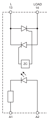
princiální schéma
