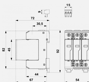
Rozměry
