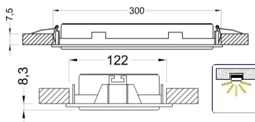
REF. REJA-BGA Anti-vandal ochranná mřížka na svítidlo
