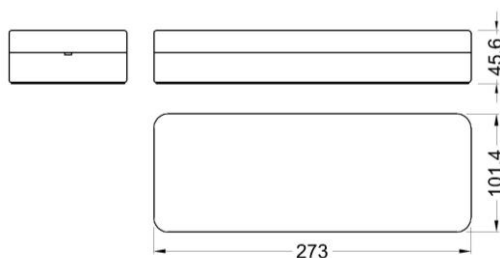
REF. AG100000 Sada pro montáž do podhledu
