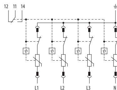
SVBC-12,5-4-MZS
