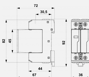
Rozměry
