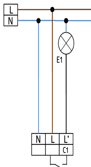
Schéma zapojení
