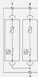
Schéma zapojení
