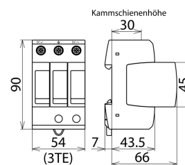
Rozměry DG M YPV SCI 1200
