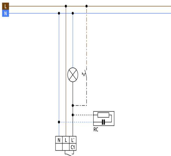
Schéma zapojení
